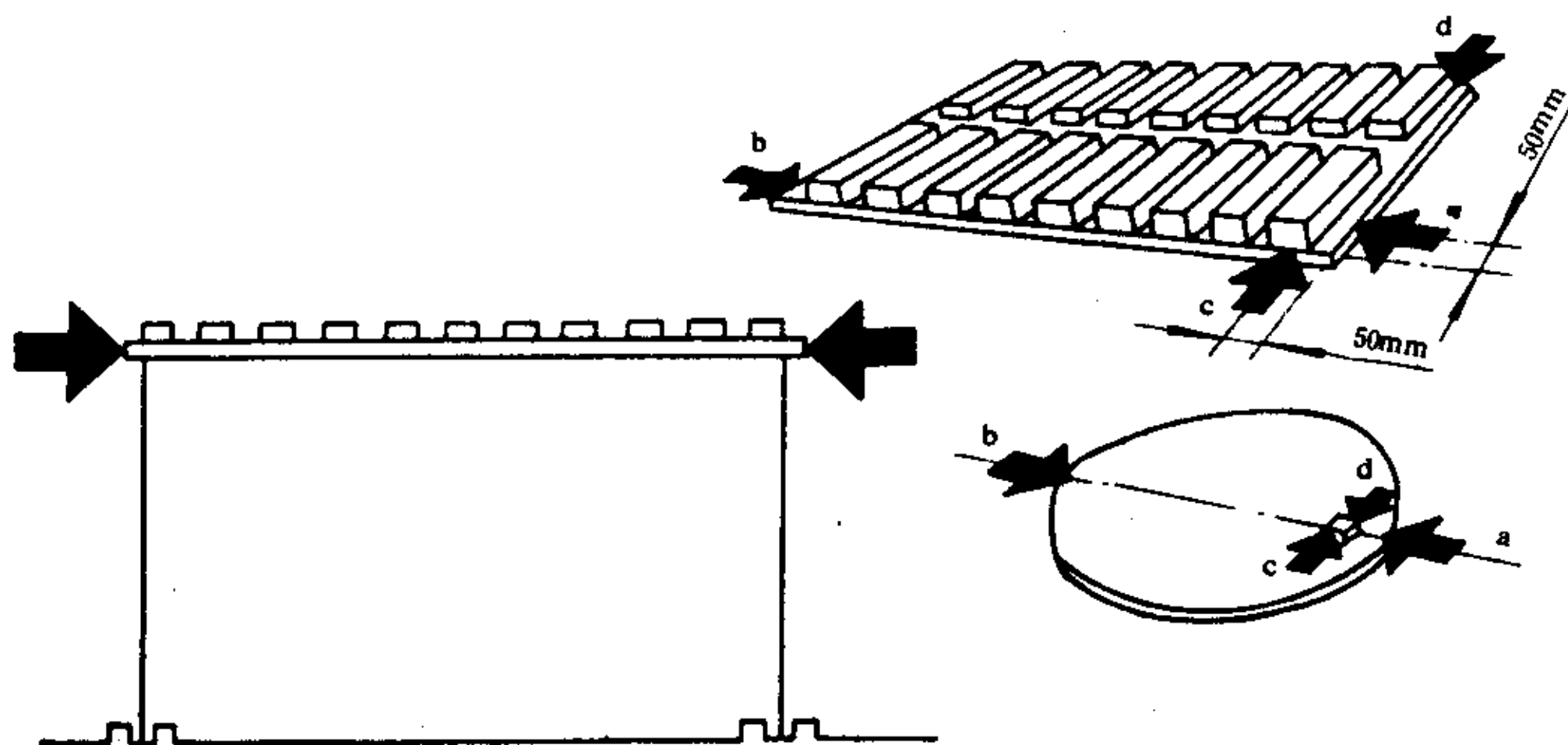
图5 桌面水平耐久性试验
