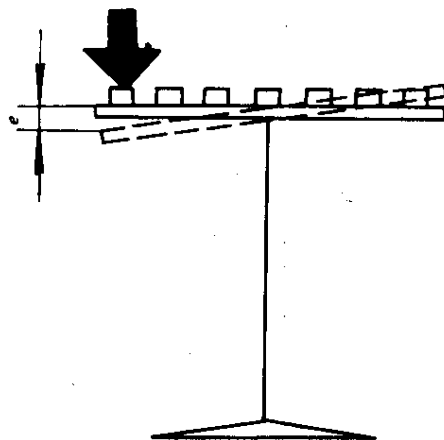
图 8 独脚桌垂直耐久性试验
