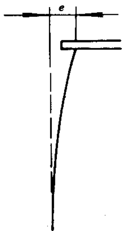
图 7 桌面水平耐久性试验位移值测量方法
