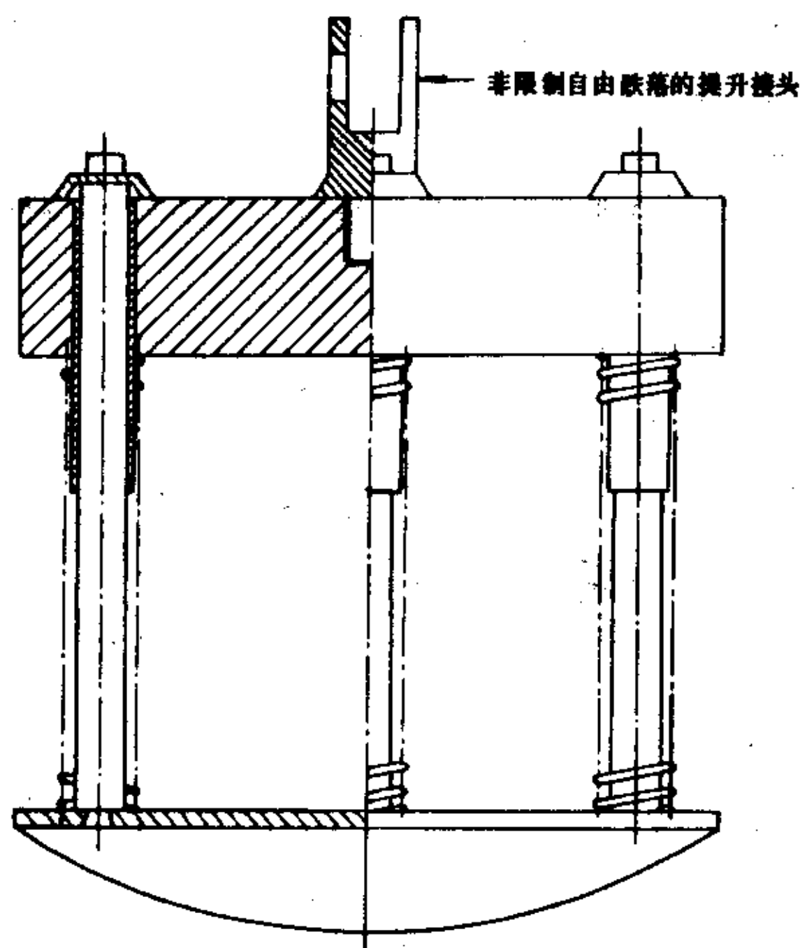
图 9 冲击器
