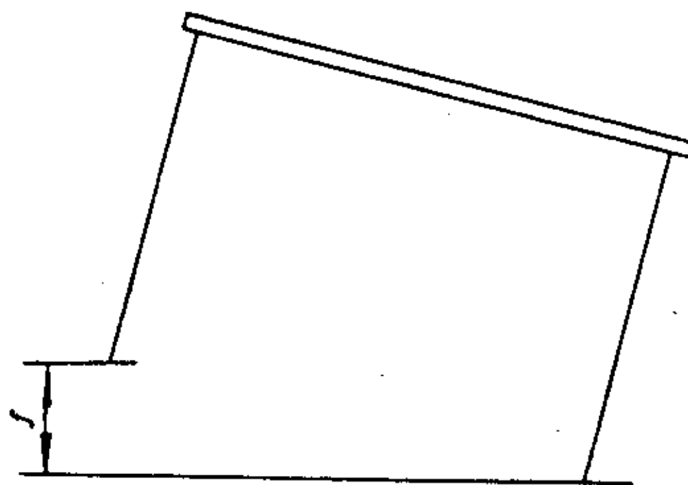
图 4 桌腿跌落试验
